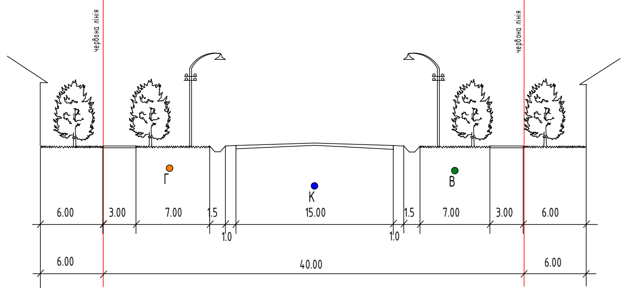
ПОПЕРЕЧНИЙ ПРОФІЛЬ 1 - 1
