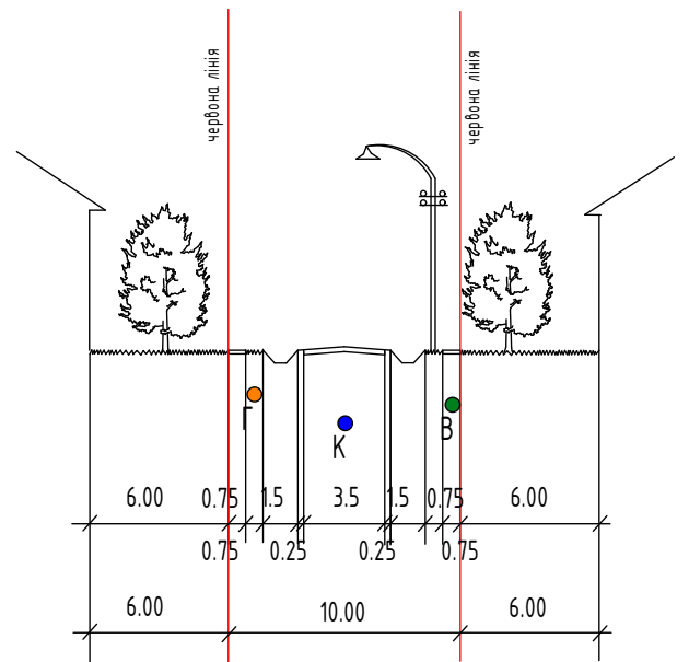
ПОПЕРЕЧНИЙ ПРОФІЛЬ 3 - 3
