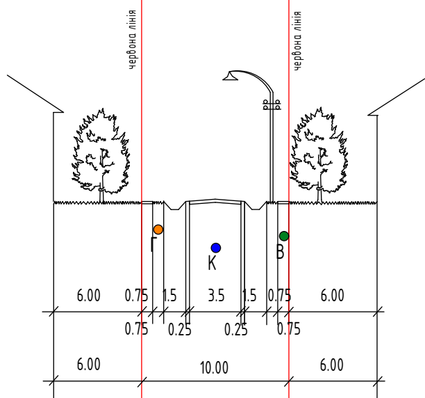
ПОПЕРЕЧНИЙ ПРОФІЛЬ 3 - 3
