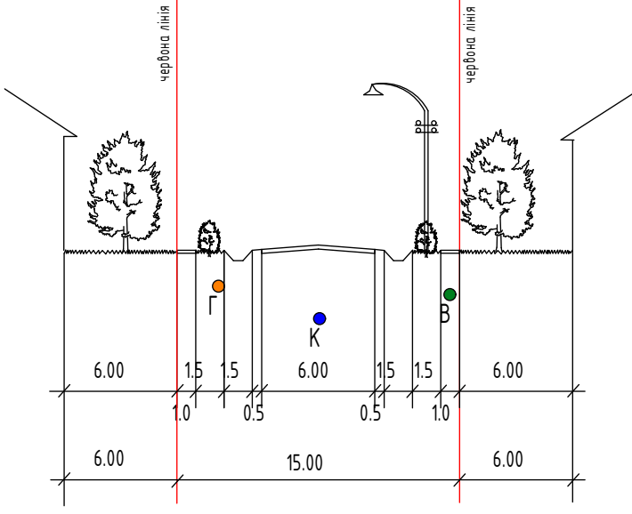
ПОПЕРЕЧНИЙ ПРОФІЛЬ 2 - 2
