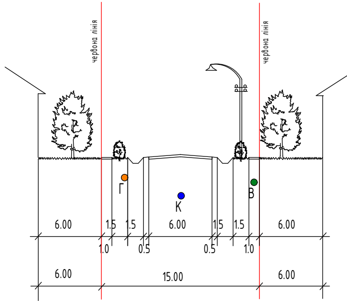
ПОПЕРЕЧНИЙ ПРОФІЛЬ 2 - 2
