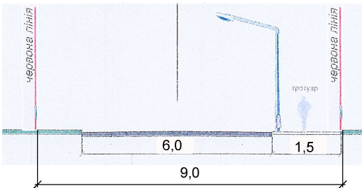
Поперечний профіль проїзду
