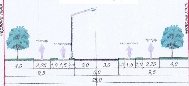
Поперечний профіль вул. Заньковецької
