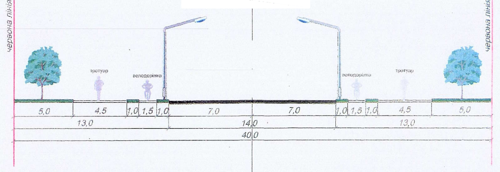
Поперечний профіль вул. Минайська, пр. Свободи
