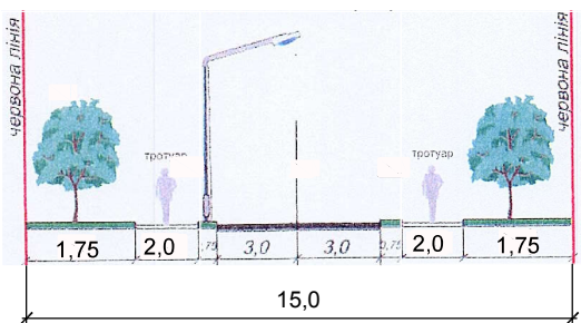
Поперечний профіль вул. 8 Березня, Проектованої
