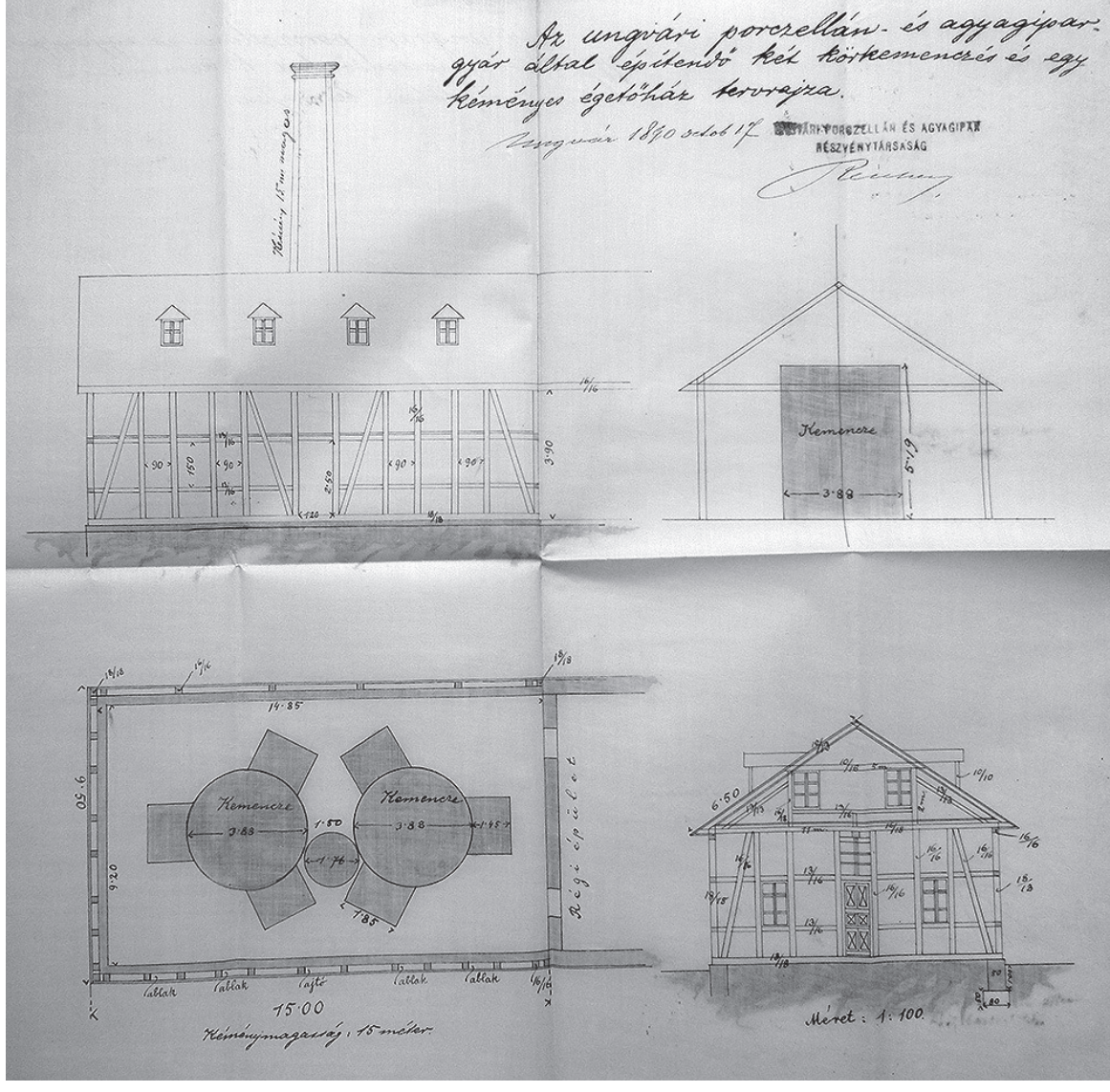
Проект будівлі, в якій розміщувалися печі для випалення продукції, 1890 рік (фонди Державного архіву Закарпатської області)
