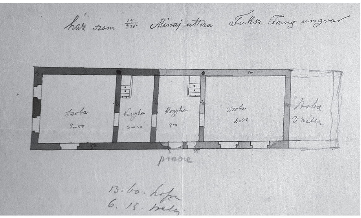
Типова забудова вулиці Минайської на прикладі будинку родини Фукс. Чорним позначено існуючу будівлю (лише одна кімната та кухня – так само було в будинку Лебовічів), сірим – запланована у 1891 році добудова. Проект – з фондів Державного архіву Закарпатської області
