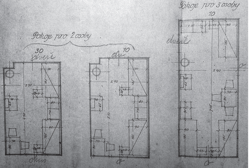
Планування кімнати для двох і трьох мешканців (із фондів Державного архіву Закарпатської області)
