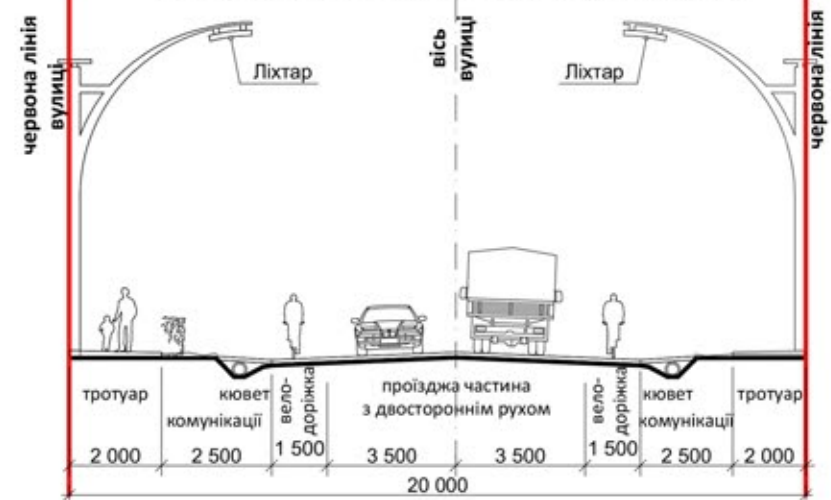
Поперечний профіль вулиці Капушанської, Володимирської та Баб'яка (1-1) М 1:200
