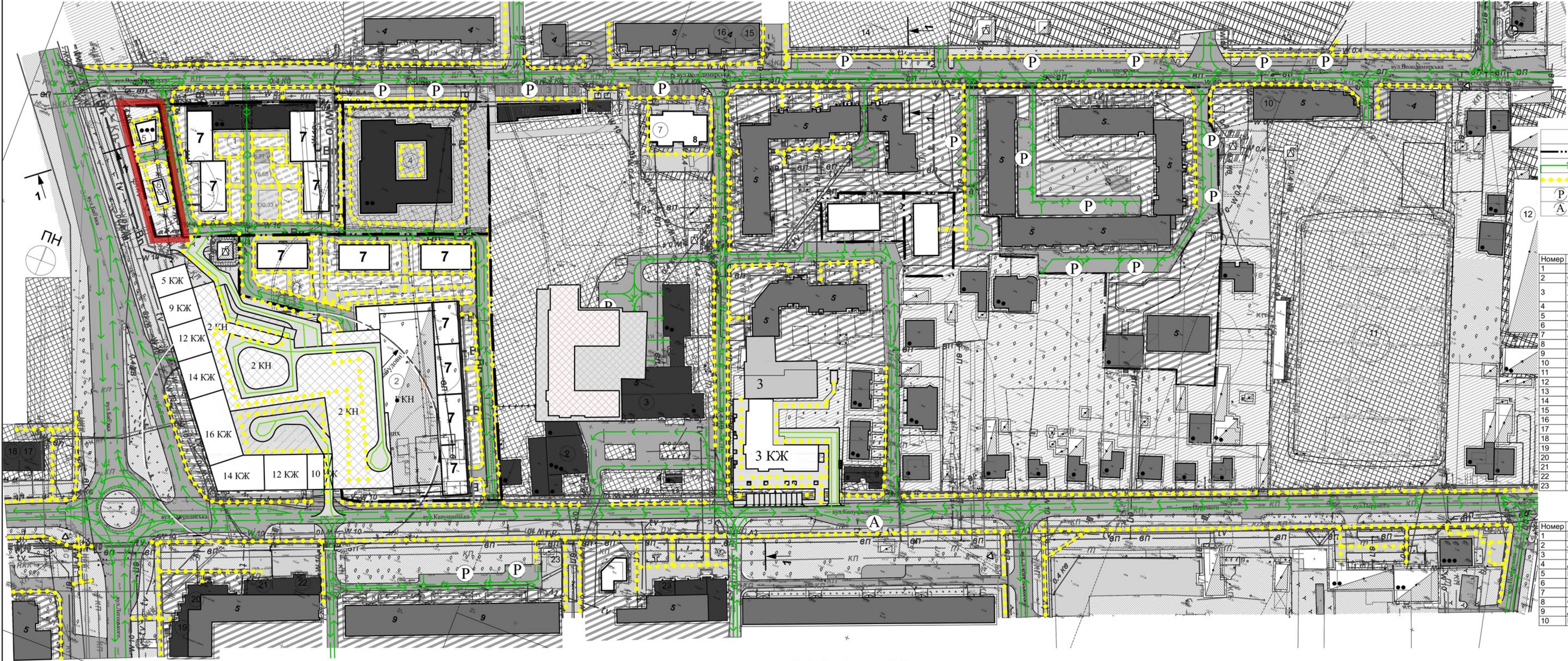
Схема організації руху транспорту і пішоходів М 1:1000
