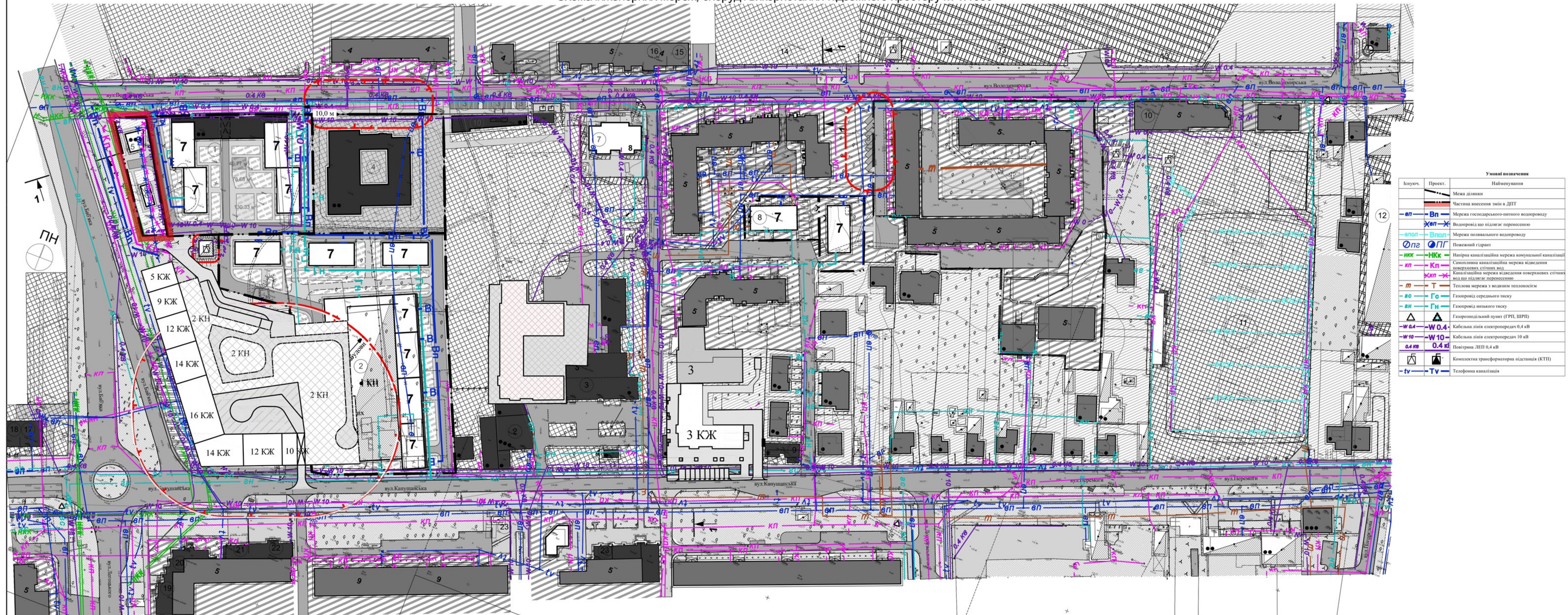
Схема інженерних мереж, споруд і використання підземного простору М 1:1000
